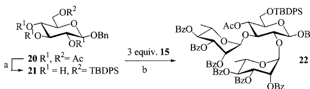
Scheme 3. a: 1) NaOMe, MeOH, 2) TPBPSCl, pyridine, DMAP, 47%; b: 1) DMTST, Et 2 O, 4-Å mol. sieves, 2) Ac 2 O, pyridine, 60%
