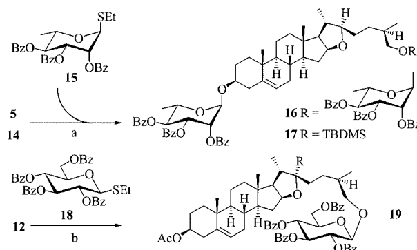
Scheme 2. a: DMTST, 4-Å mol. sieves, Et 2 O, argon, 6 h, room temp.; b: DMTST, 4-Å mol. sieves, CH 2 Cl 2 , argon, 4.5 h, room temp.
